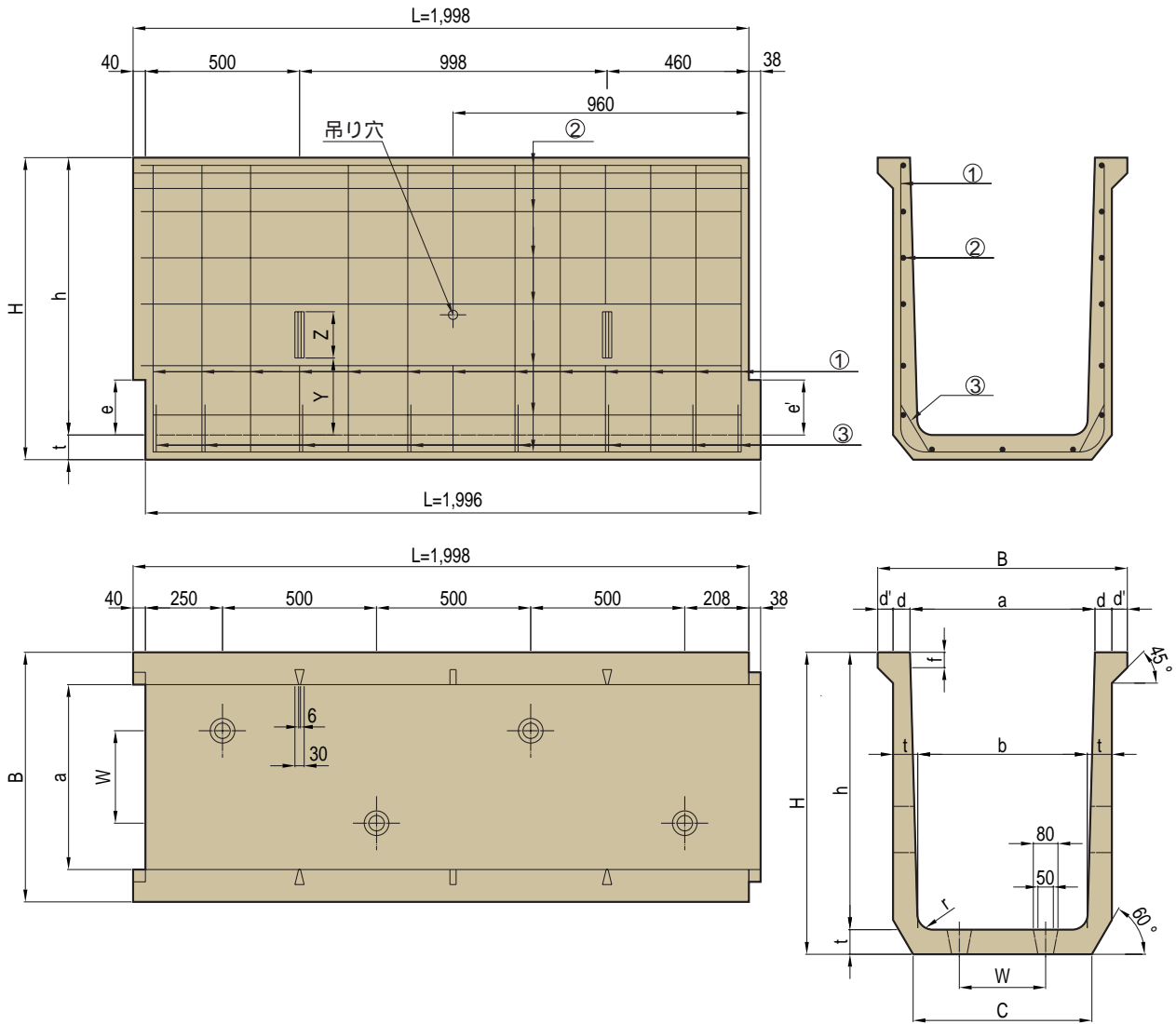
排水フリューム形状寸法及び配筋表
